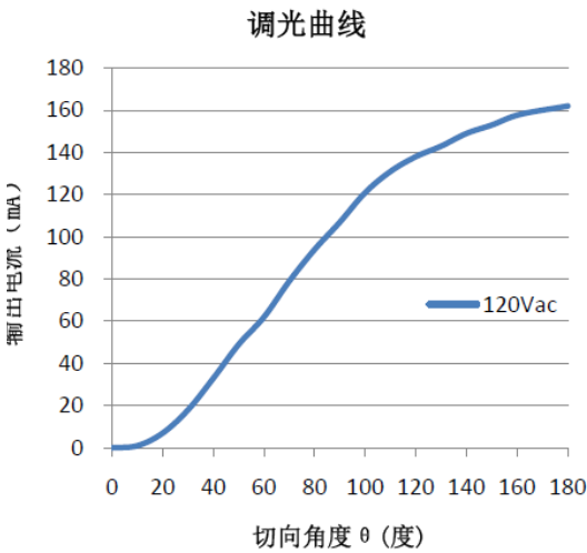
MT7893 调光曲线
