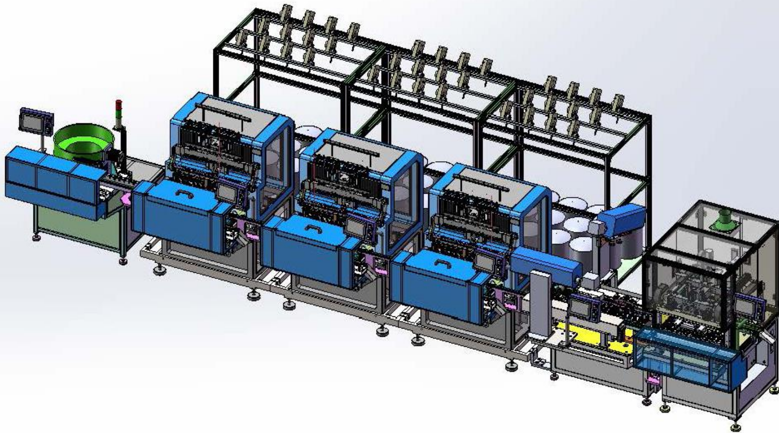
自动上料机+N台绕线机+激光脱皮机+焊锡机
