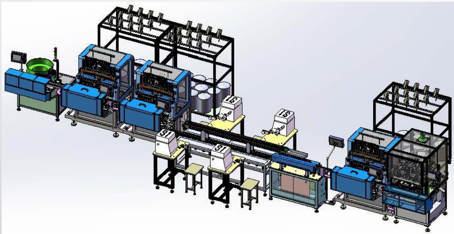
自动上料机+N台绕线机+铜箔工位+激光脱皮机+焊锡机
