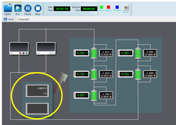
ITS5300测试系统截图——均充均放
